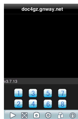
Hình 1 Menu Chính
